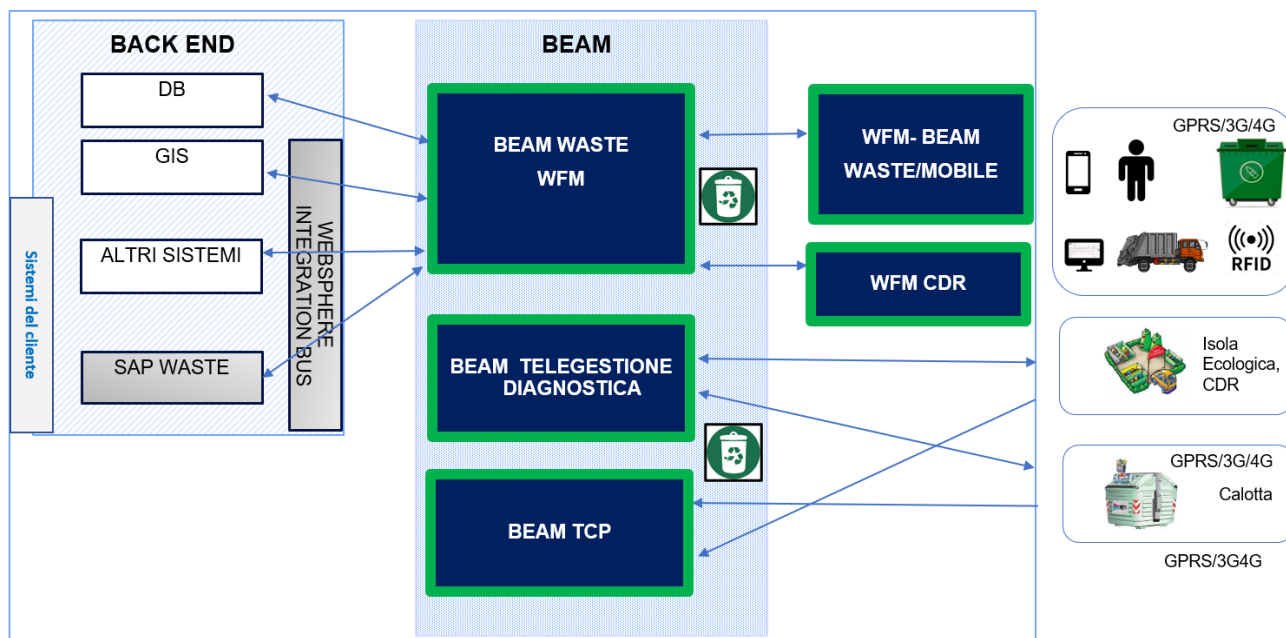
Figura 2. Macro Architettura della componente BEAM IoT Waste.
