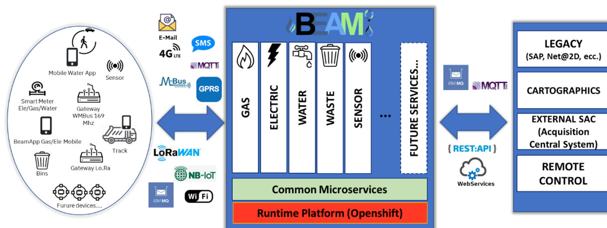
Figura 1. Macro Architettura della soluzione: esempi di protocolli supportati, moduli verticali disponibili e integrazione con sistemi esistenti.
