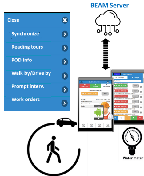
Figura 4. Esempi di funzionalità BeamApp Idrico – Walkby/Driveby.
