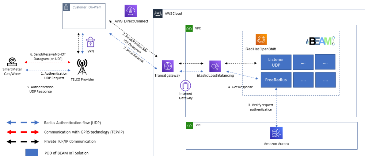
Figura 10. Flusso di autenticazione tramite APN privato e tecnologia di comunicazione NB-IoT e protocollo UDP. In questo caso è previsto il passaggio dalla rete on-prem.
