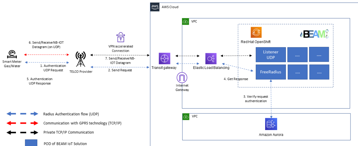
Figura 9. Flusso di autenticazione tramite APN privato e tecnologia di comunicazione NB-IoT e protocollo UDP.
