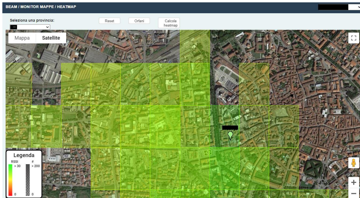
Figura 6. Esempio di funzione BEAM IoT per la copertura WMBus 169 MHz rappresentata su Heatmap.
